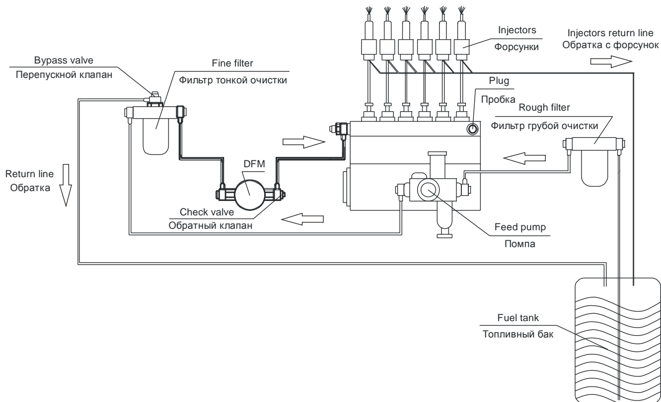
Рис. 3 Установка DFM на давление
