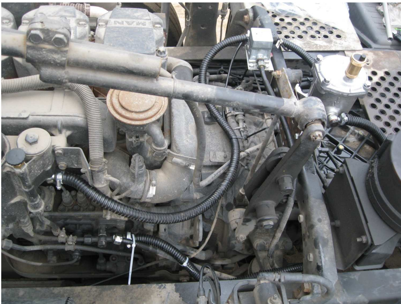
Рис. 6 Схема установки DFM на разрежение с деаэратором на двигатель MAN
